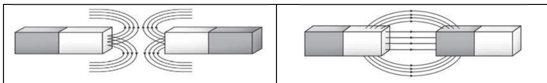
Gambar 7. Garis medan magnet antara dua kutub magnet senama dan tidak senama
