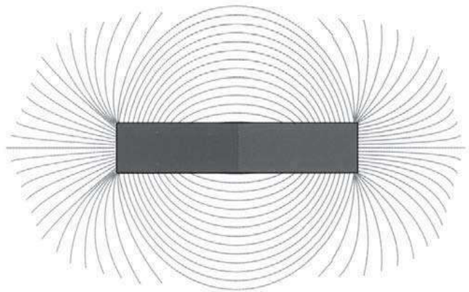
Gambar 6. Gaya paling kuat terletak pada kutub magnet
