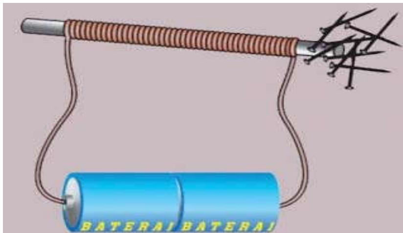
Gambar 5. Magnet dengan cara Elektro Magnet
