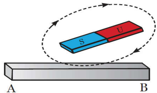
Gambar 3. Magnet dengan cara digosok
