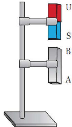
Gambar 4. Magnet dengan cara induksi
