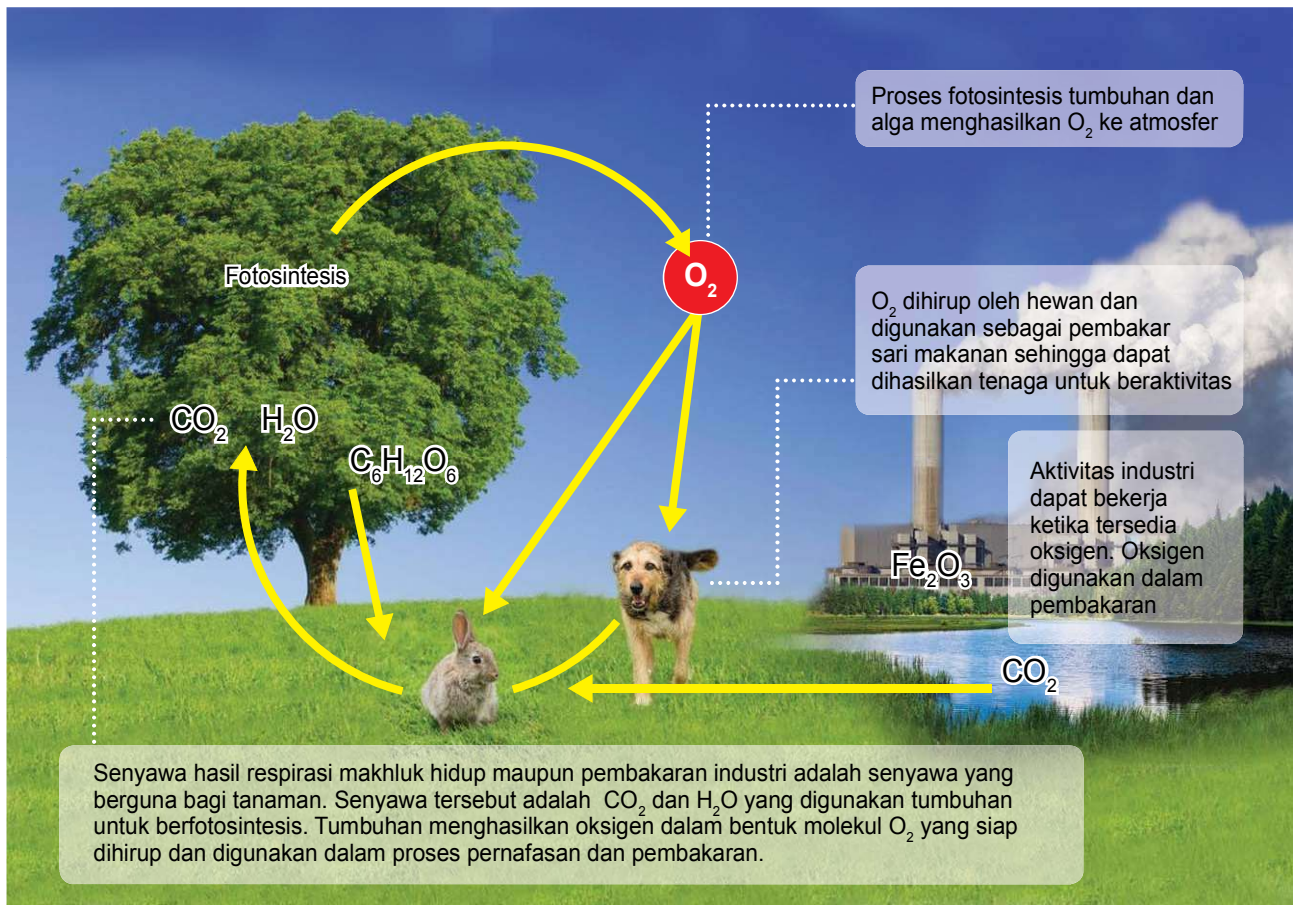
Gambar 8. Daur oksigen
